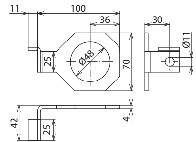
Maßbild AB EXFS IF1 W 48
