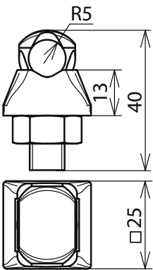
Maßbild KSV 6.10 FER CU
