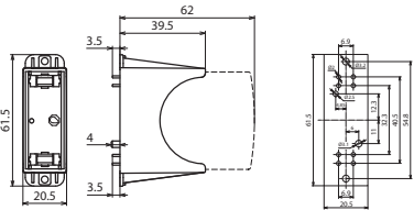
Maßbild DG PCB PV SCI 600
