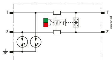
Prinzipschaltbild BCO MOD ML2 BD HF 5
