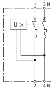
Prinzipschaltbild POP 2 255 C25
