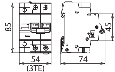
Maßbild POP 2 255 C25
