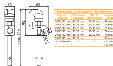
Maßbild UK 25 SQL
