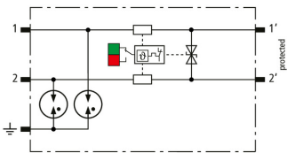
Prinzipschaltbild BCO CL2 BD 12
