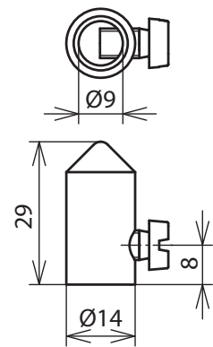
Maßbild FS 8 MSGALCU
