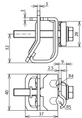
Maßbild DRK KB 8.10 W16.22 EST STTZN
