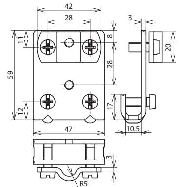
Maßbild FK ZS 7.10 KBF0.7 10 STTZN
