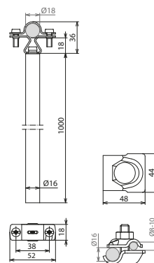
Maßbild DH PAE 18 D16 1000 AL V2A
