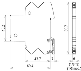
Maßbild BCO CL2 E 24
