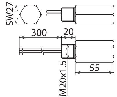
Maßbild DPI CD HF EXD 5 M
