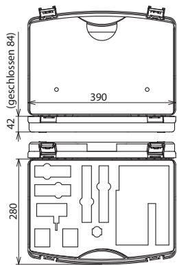
Maßbild KKL DCA
