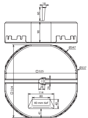
Maßbild BES 17KG KT16 ULP D337 SET
