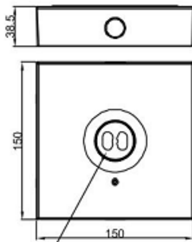
Asymmetrische Linse für Rettungswege | asymmetric lens for escape routes
