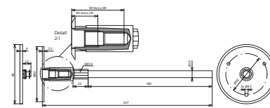
Maßbild EFPM M10 12 V4A L245 VP STTZN
