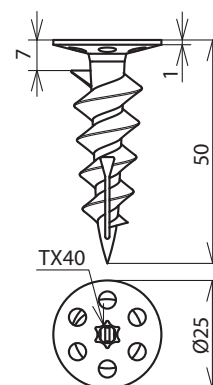
Maßbild HSPD HS4.5 L50 PA
