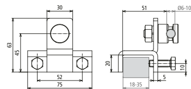
Maßbild AK 6.10 KSV FER S KBF18 35 V2A
