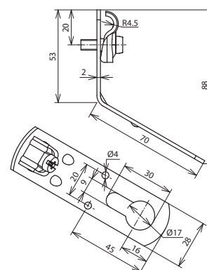
Maßbild DLH DQ 6.10 WPRO5 8 STTZN
