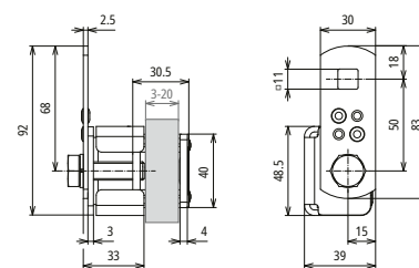
Maßbild AKK AL B11.11 KBF 3 20 STTZN
