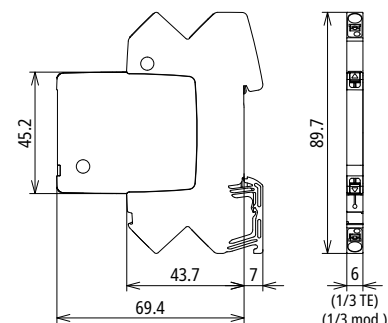
Maßbild BCO ML2 BD 180
