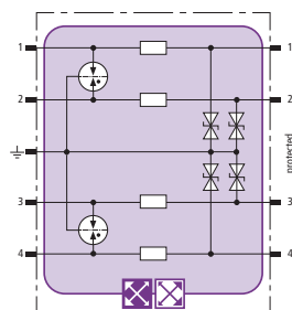
Prinzipschaltbild BXT ML4 BE 60
