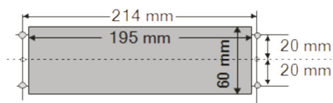
Masszeichnung Einbau- / Unterputzkasten
