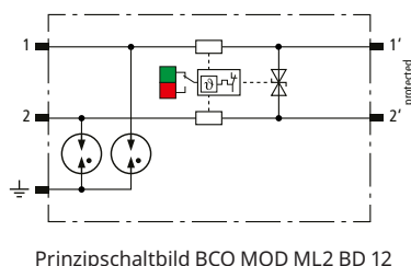
Prinzipschaltbild BCO MOD ML2 BD 12
