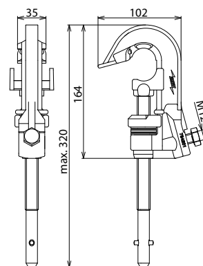
Maßbild PSK 4 30 SQL
