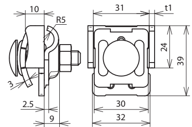
Maßbild FK KB 6.10 KBF0.7 8 STTZN
