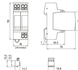
Maßbild DG MP TT 2P ACI 385 FM
