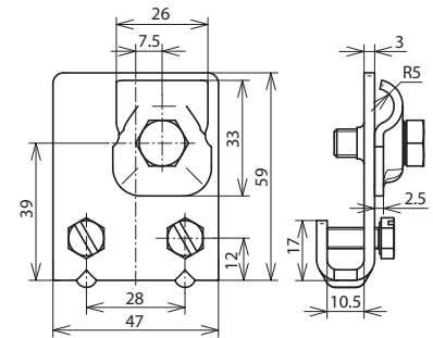
Maßbild FK KB 6.10 KBF0.7 10 CU
