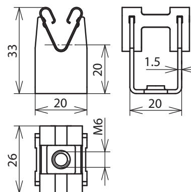
Maßbild LH DG 8 H20 IGM6 V2A
