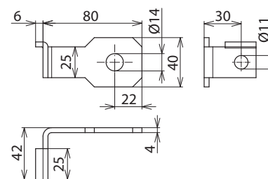
Maßbild AB EXFS IF1 W 14
