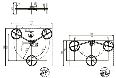
Maßbild DBS KB D40.50 RA620 STTZN
