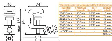
Maßbild UEK 30 SKN
