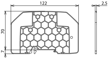
Maßbild PARTITION EXI
