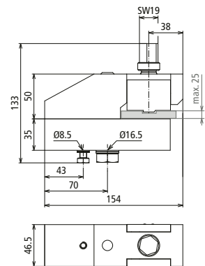
Maßbild KLFP M16 KSS
