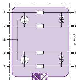
Prinzipschaltbild BXT ML4 BD 5
