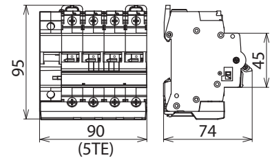
Maßbild POP 4 255 C32
