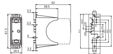
Maßbild DG PCB NPE FM
