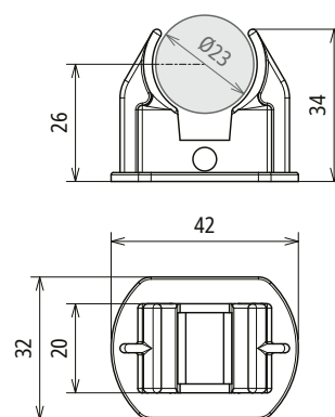
Maßbild RLA 23 FB K SW
