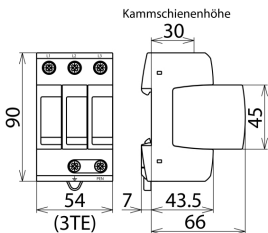
Maßbild DG M TNC 385
