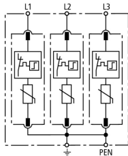
Prinzipschaltbild DG M TNC 385
