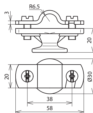
Maßbild LH ZS 13 IGM8 STTZN ZG
