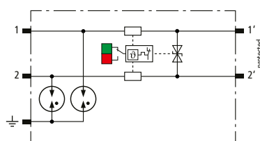
Prinzipschaltbild BCO ML2 BD 48
