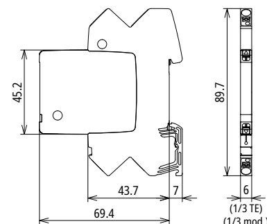
Maßbild BCO ML2 BD 48
