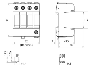
Maßbild DG MD TT ACI 275 FM
