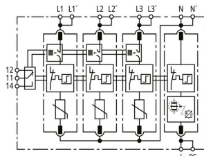
Prinzipschaltbild DG MD TT ACI 275 FM
