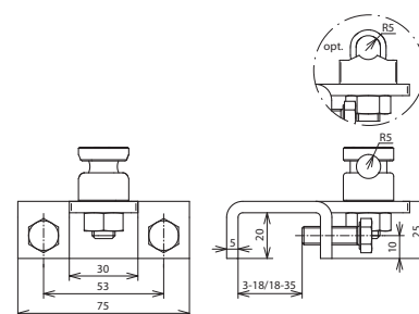
Maßbild AK 6.10 KSV W KBF3 18 V2A
