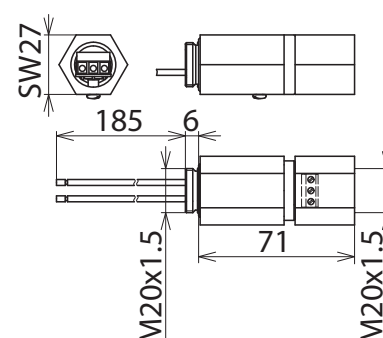
Maßbild DPI MD 24 M 2S
