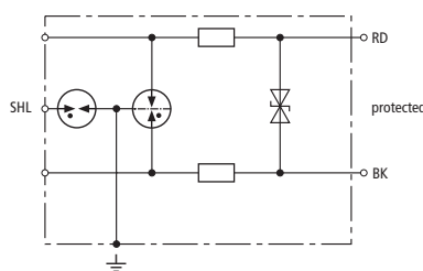
Prinzipschaltbild DPI MD 24 M 2S
