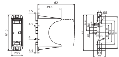
Maßbild DG PCB PV I 500 FM
