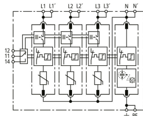
Prinzipschaltbild DG MP TT ACI 385 FM
