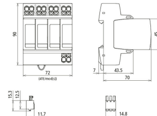
Maßbild DG MP TT ACI 385 FM
