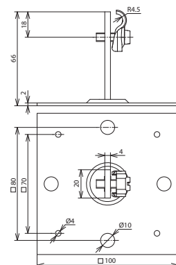
Maßbild DLH DQ 6.10 GP100X100 STTZN
