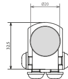
Maßbild
