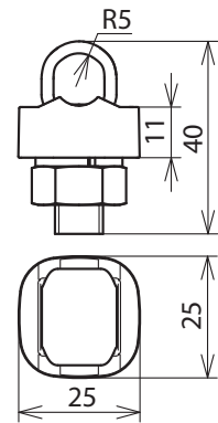
Maßbild KSV 7.10 FER STTZN
